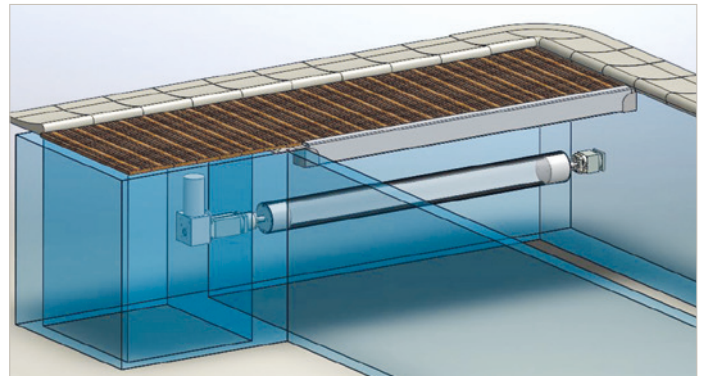
› Coupe moteur en fosse sèche : principe d'intégration
